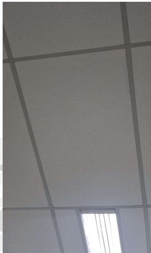
Imagem 4: Detalhe do layout da instalação da placa de forro de gesso com recorte da luminária
